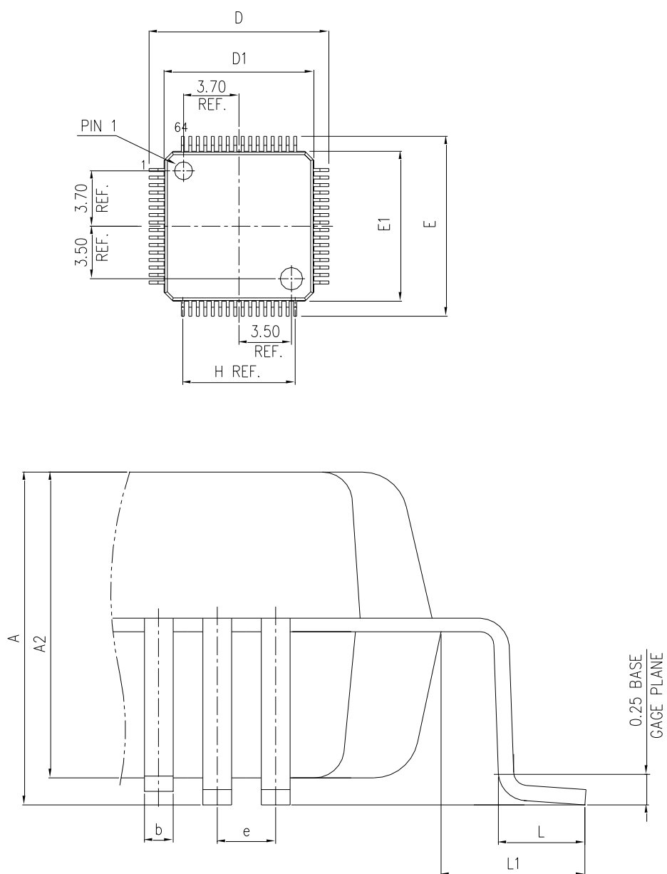
图 20 LQFP64 封装图
