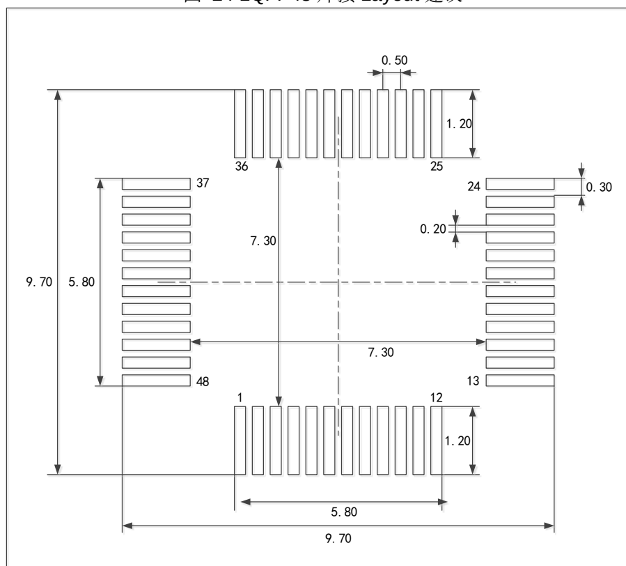
图 24 LQFP48 焊接 Layout 建议
