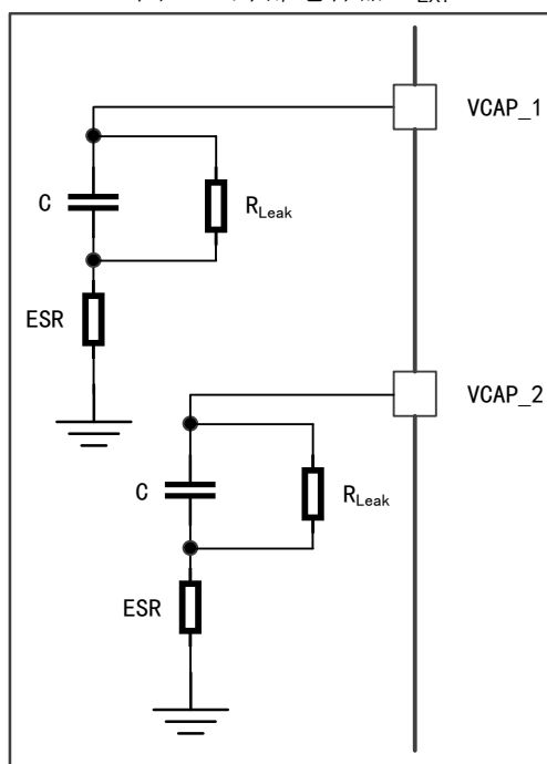
图 11 外部电容器 C_{EXT}
