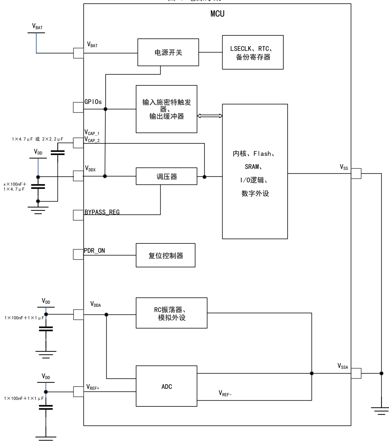
图 7 电源方案
