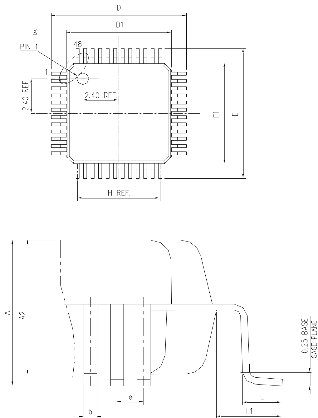
图 23 LQFP48 封装图
